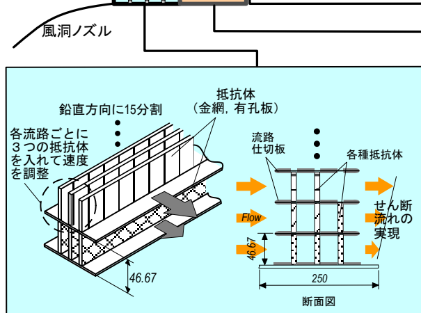
速度成層形成装置： 様々な速度分布を持つ流れ場を形成できる
