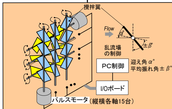
乱流発生装置： 大気乱流に相似した乱流場の形成が可能
