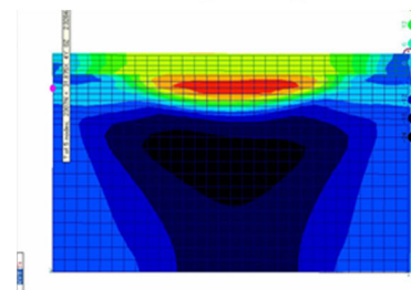
図3 残留応力分布の予測
