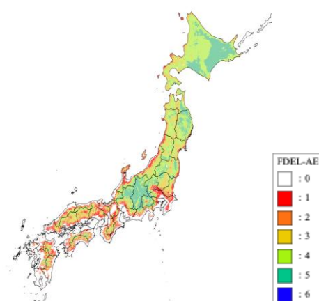
AE コンクリートを想定した凍害地域性評価結果
