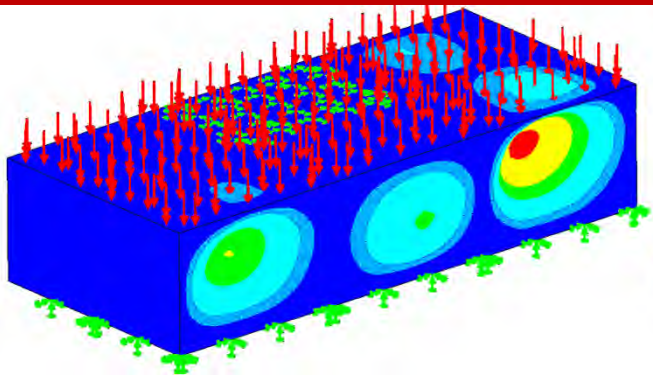
コンピュータで機械的強度を解析
